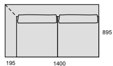
FOX 2-KRESLO-1P 1595 x 895 / 710
